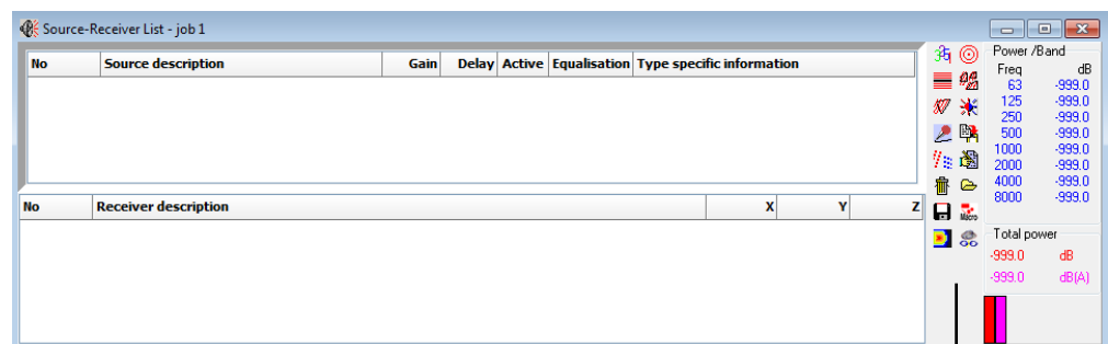
Local Toolbar
